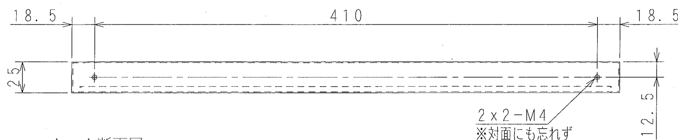
A-A断面図
