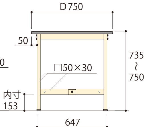
側面図
