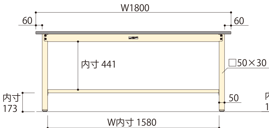
正面図
