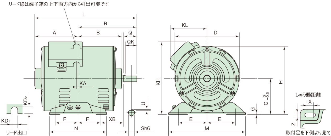
外形寸法表 (mm) 50/60Hz 100V
