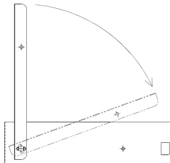
組立要領図
