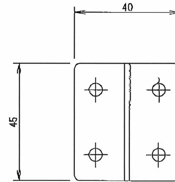
B. へり付き金具
