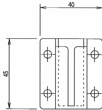
A. 受け金具
