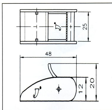
バックル寸法
