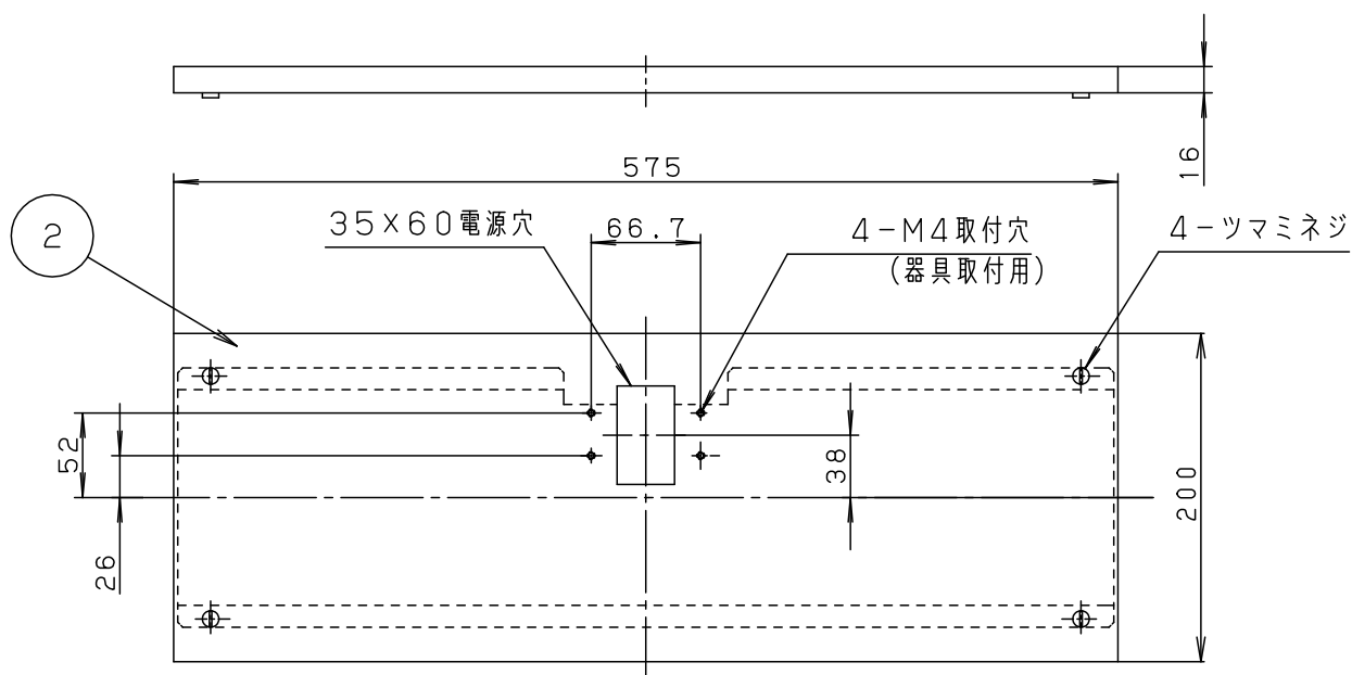
背面図
