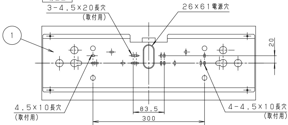
背面図
