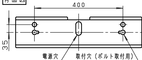
背面図
