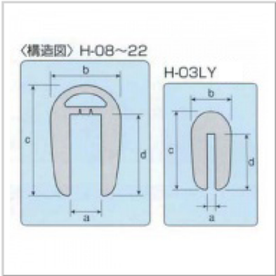
構造図
