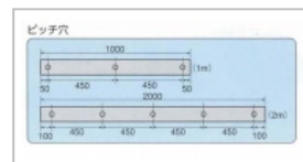
ピッチ穴
