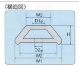
構造図
