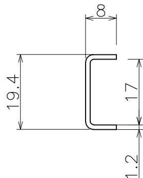
製作治具断面図
