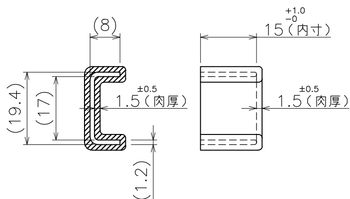
製品図
