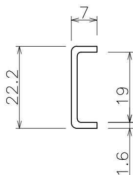
製作治具断面図
