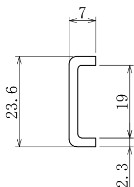
製作治具断面図
