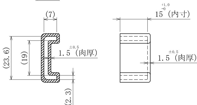
製品図
