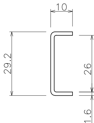
製作治具断面図
