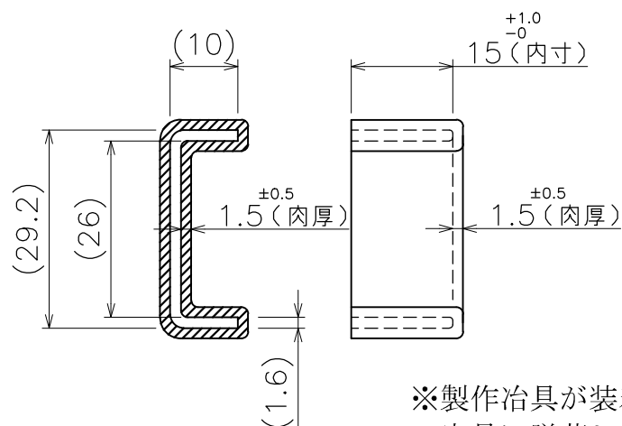
製品図
