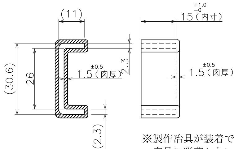
製品図
