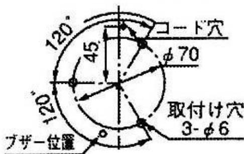
取付面寸法図
