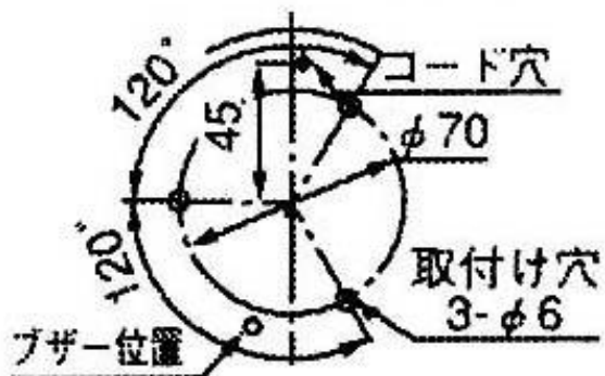
取付面寸法図
