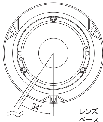
底面図
