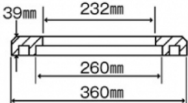
断面図
