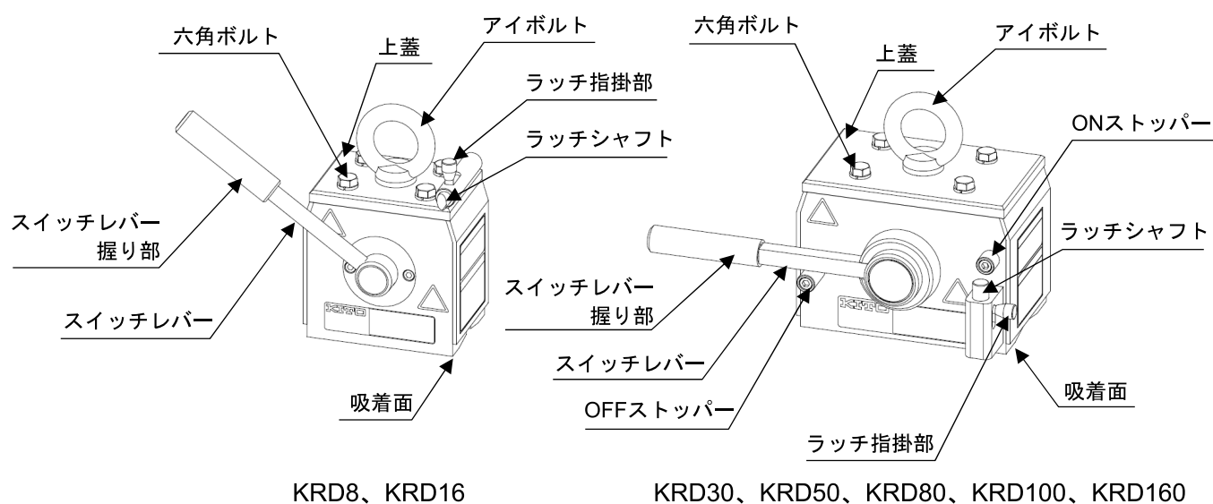
図1-1 各部の名称
