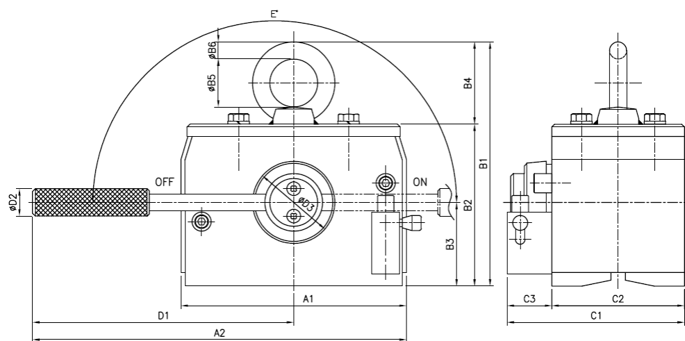
图4-3 KRD30、KRD50、KRD80、KRD100、KRD160的外形图
