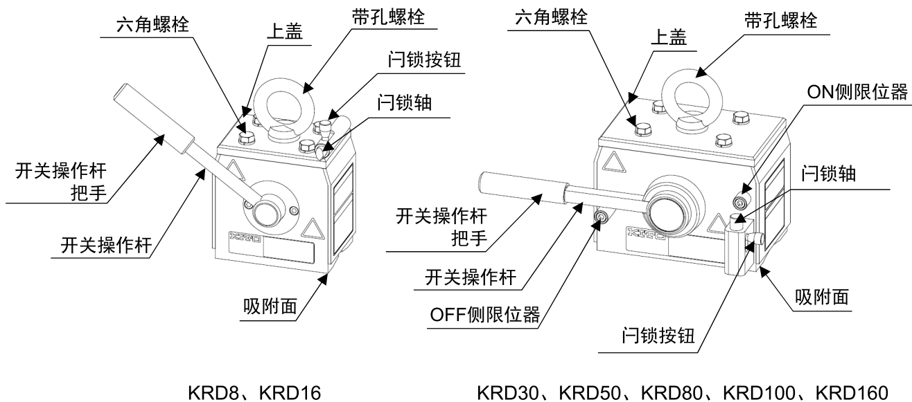
图1-1 各部的名称
