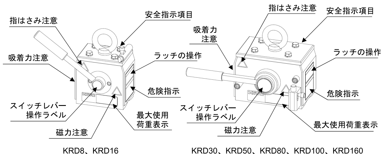
図1 本体の表示
