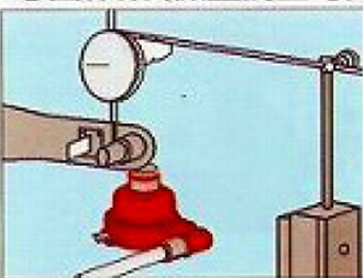
芯出作業（微量調整可）
