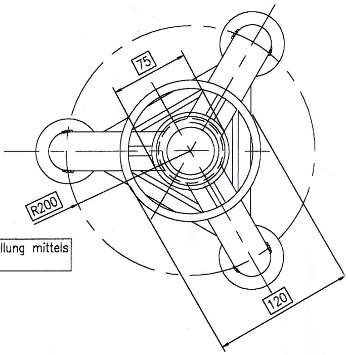
Draufsicht ohne Gewindestempel gezeichnet.
