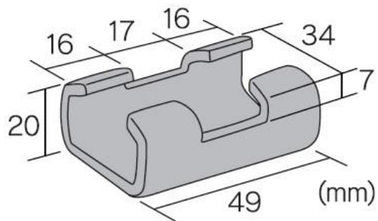
サドル部寸法
