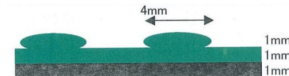
※1) 断面図(EA997RA-13)
