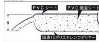
断面形状
