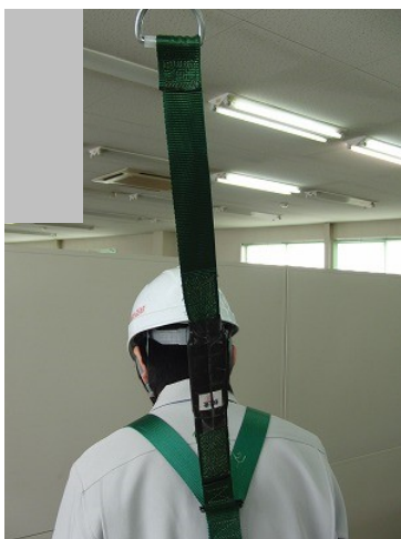
⑤落下を阻止したときの荷重に応じてショックアブソーバが展開する。
