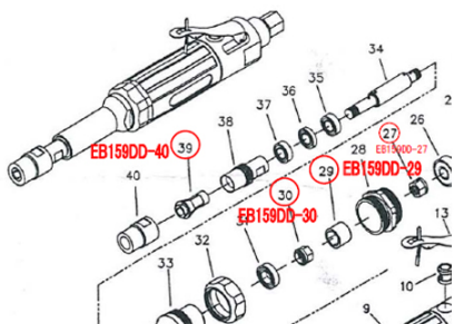
NO.27 カップリングナット
